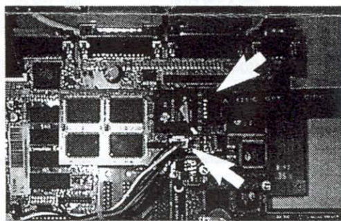
ABBILDUNG 2: HIER IST DAS CONNECT-MODUL AN DIE BVISIONPPC ANGESCHLOSSEN, SOWIE DAS FLOPPY-STROMVERSORGUNGSKABEL – VOM NETZTEIL KOMMEND – AUF DEN A1200-FLOPPY-STROMSTECKER AUFGESTECKT.
