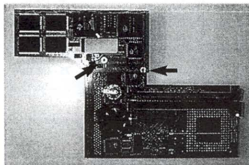
ABBILDUNG 1: IN DIESER AUSRICHTUNG WIRD DIE BVISIONPPC AUF DER BLIZZARD603E/E+ AUFGESTECKT.
