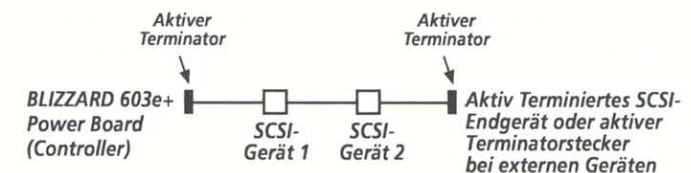
Bild 10. Beispiel einer SCSI-Gerätekette mit korrekt gesetzten aktiven Terminatoren
