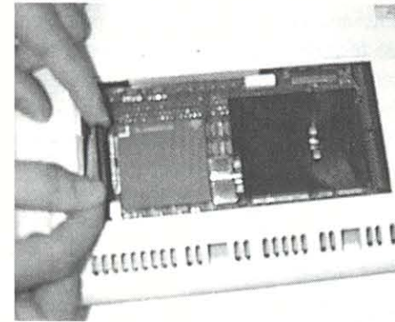
Bild 5. Aufstecken des 50poligen SCSI-Steckers
